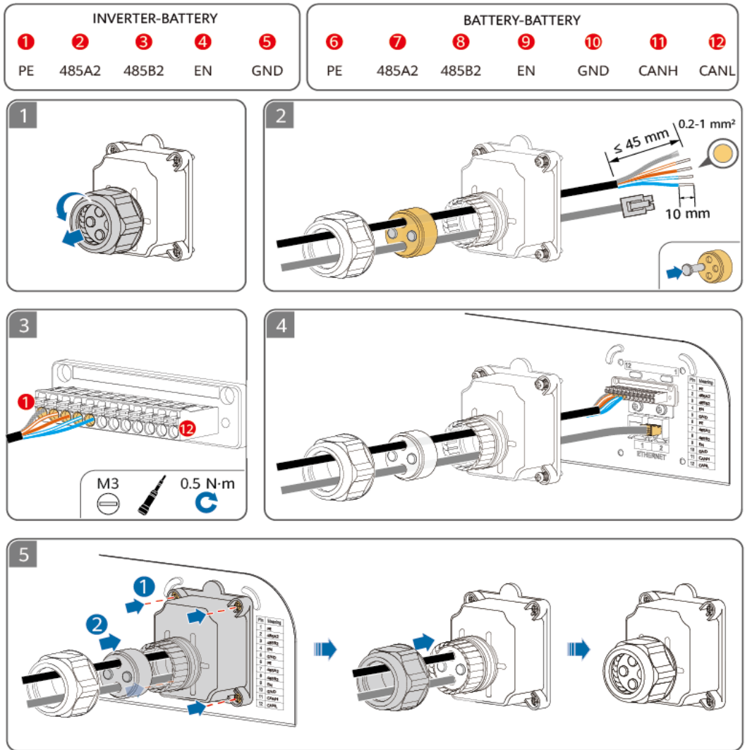
Abbildung 5-7 Signalanschlussverbindungen
