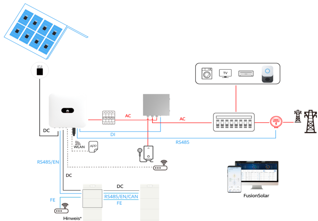
Abbildung 2-8 Netzgekoppeltes/-entkoppeltes Szenario
