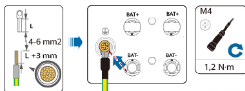
Abbildung 5-3 Anschließen des PE-Kabels
